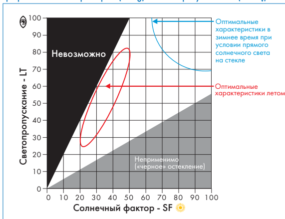
График: Солнечный фактор SF (или g) — Светопропускание LT (или \tau_v )
