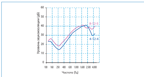
Спектр звукоизоляции для однокамерных стеклопакетов в конфигурации 4-12-4 и 8-12-5
