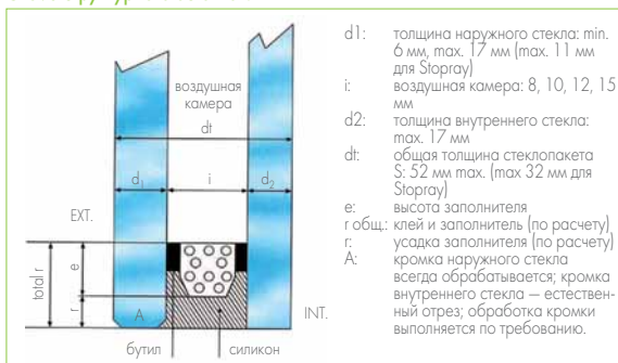
Схема структурного остекления
