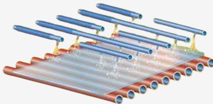
РИС. [2]: РАСПРЕДЕЛЕНИЕ ГОРЯЧЕГО ВОЗДУХА ПО ВЕРХНЕЙ ПОВЕРХНОСТИ СТЕКЛА
